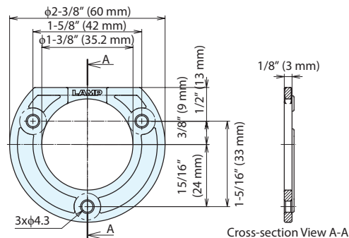
[Spacer]
